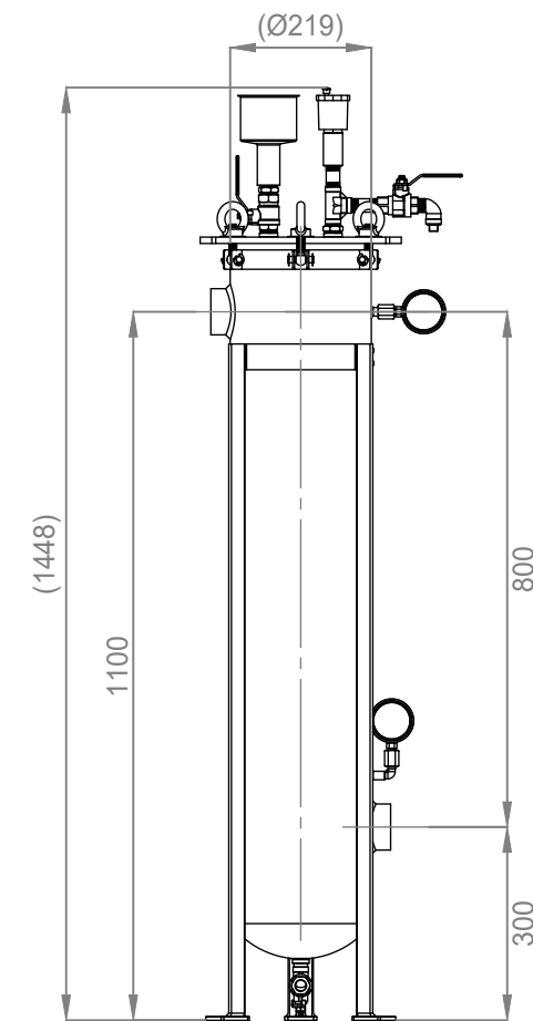
GLF-50-LT
