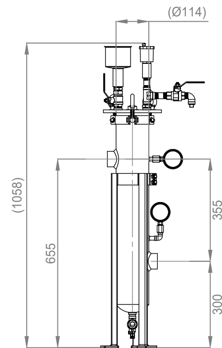
GLF-32-LT
